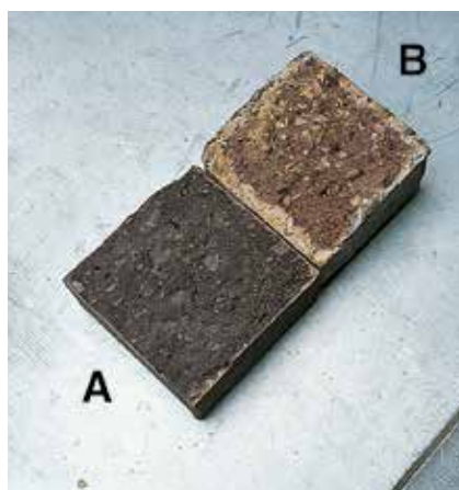
Fot. 1. Próba penetracji jonami chloru (UNI 9944). Próbka A została zabezpieczona izolacją Mapelastic i nie wykazuje penetracji; próbka B, bez izolacji wykazuje zniszczenia różnej wielkości.
