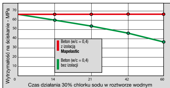
Rys. 4 Wpływ izolacji Mapelastic na ograniczenie spadku wytrzymałości betonu spowodowanego działaniem soli ołdziejających, zawierających chlorek wapnia.
